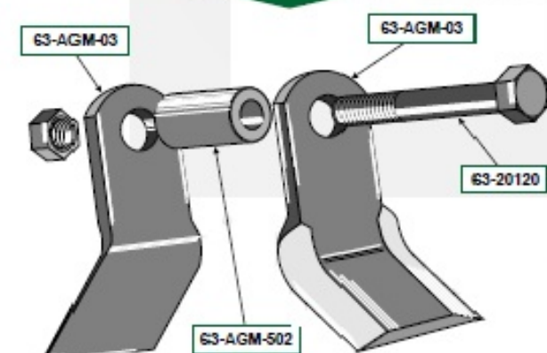
Anzahl der Y-Messer, Buchsen und Schrauben nombre de couteaux-Y, entretoises et boulons number of Y-Blades, bushes and bolts
