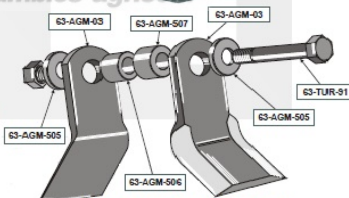
Anzahl der Y-Messer, Buchsen und Schrauben nombre de couteaux-Y, entretoises et boulons number of Y-Blades, bushes and bolts
